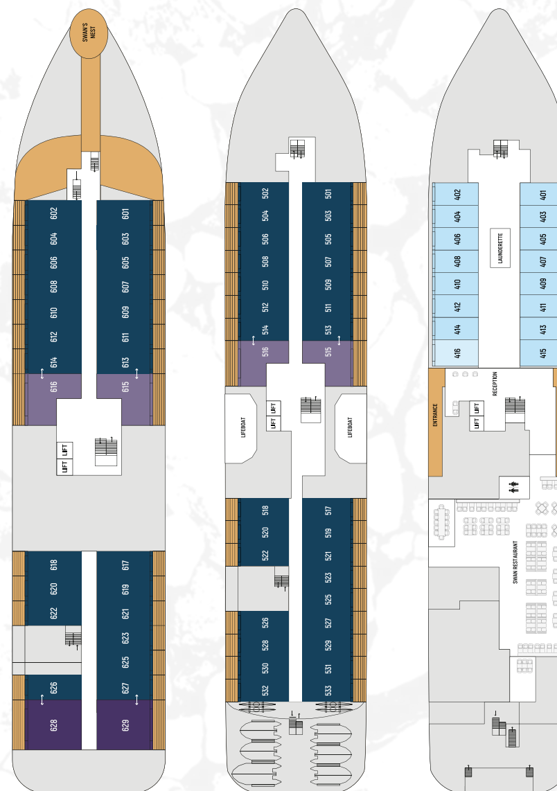
Палуба 6
